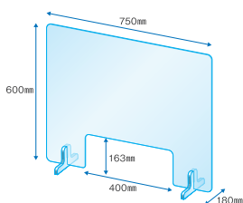
NCW-2 (W750mm×H600mm)
