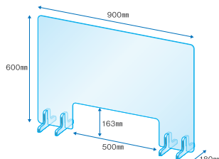
NCW-3 (W900mm×H600mm)
