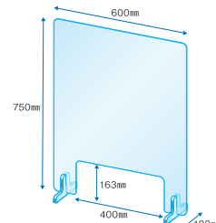
NCW-1H (W600mm×H750mm)
