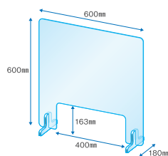
NCW-1 (W600mm×H600mm)
