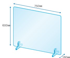
NC-2 (W750mm×H600mm)
