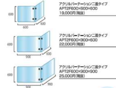
●アクリル板(透明)・厚さ3mm~4mm ※サイズにより異なります ●金具=アルミ押出し アルミマウント上(シルバー)
