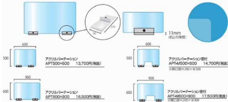
●アクリル板(透明)・厚さ3mm~4mm ※サイズにより異なります ●ベース部=材質:スチール製鋼(SPHC) 表面処理:焼付け塗装(白色)
