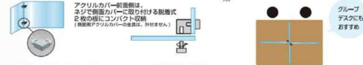
●アクリル板(透明)・厚さ3mm~4mm ※サイズにより異なります ●金具=アルミ押出し アルミマウント上(シルバー)
