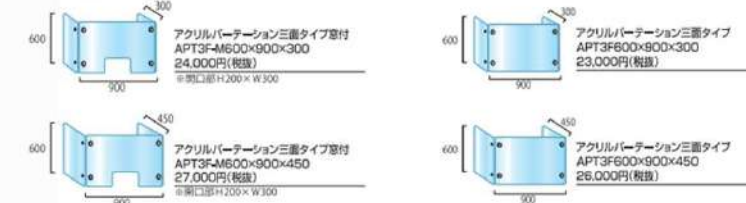
●アクリル板(透明)・厚さ3mm~4mm ※サイズにより異なります ●金具=アルミ押出し アルミマウント上(シルバー)
